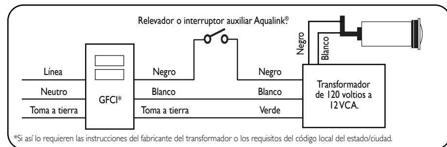
Figura 5: Cableando las luces subacuáticas VÜ LED sin nicho .
